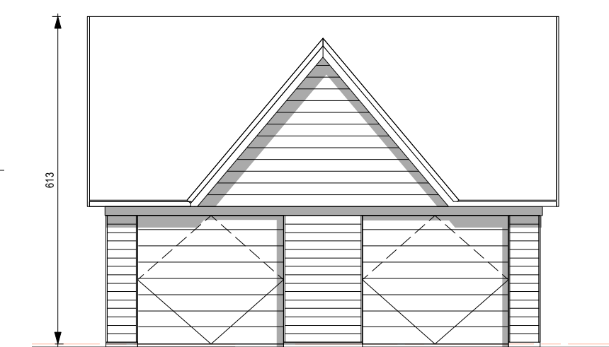
Voorgevel garage
