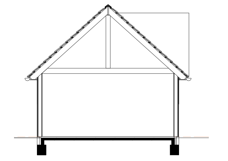
Doorsnede garage
