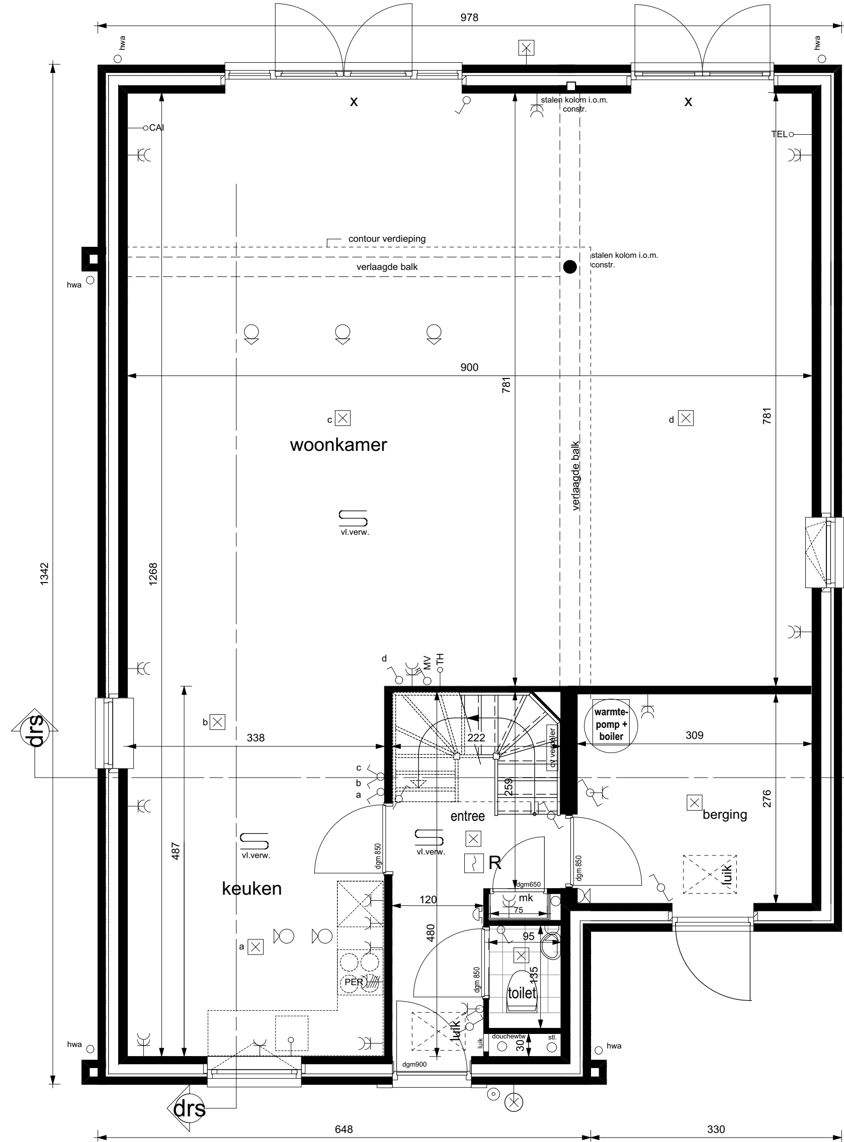
Begane Grond
