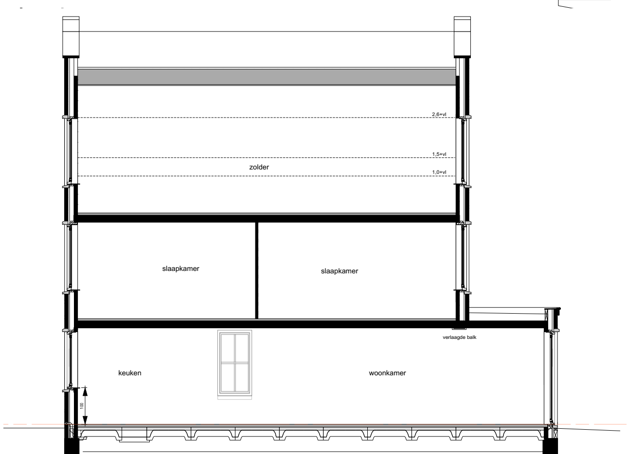
Doorsnede
