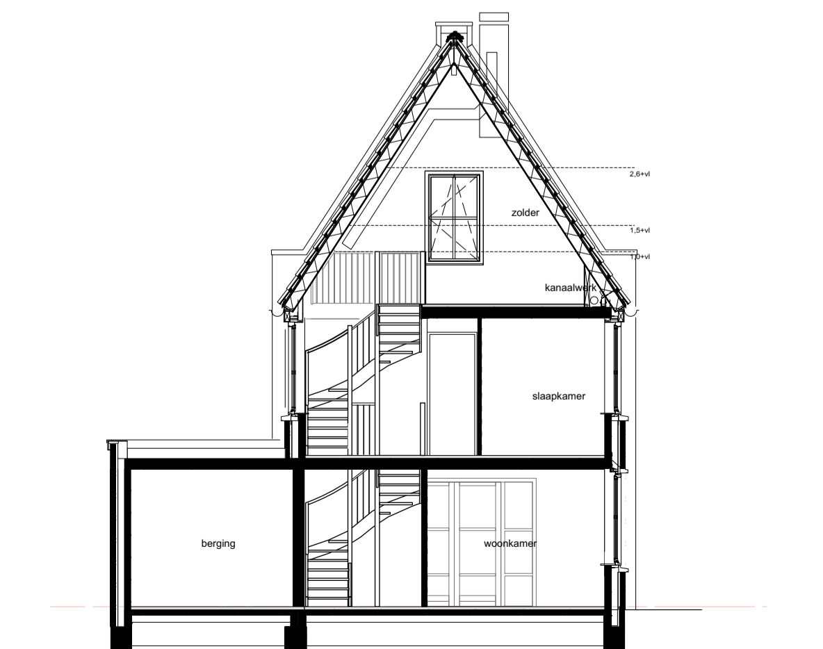
Doorsnede
