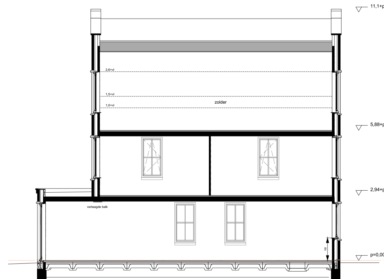
Doorsnede
