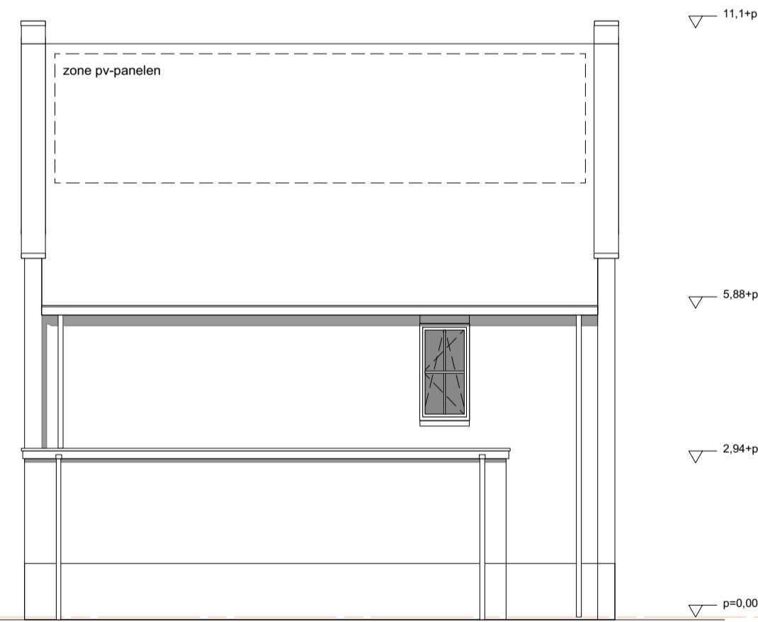
Zijgevel links
