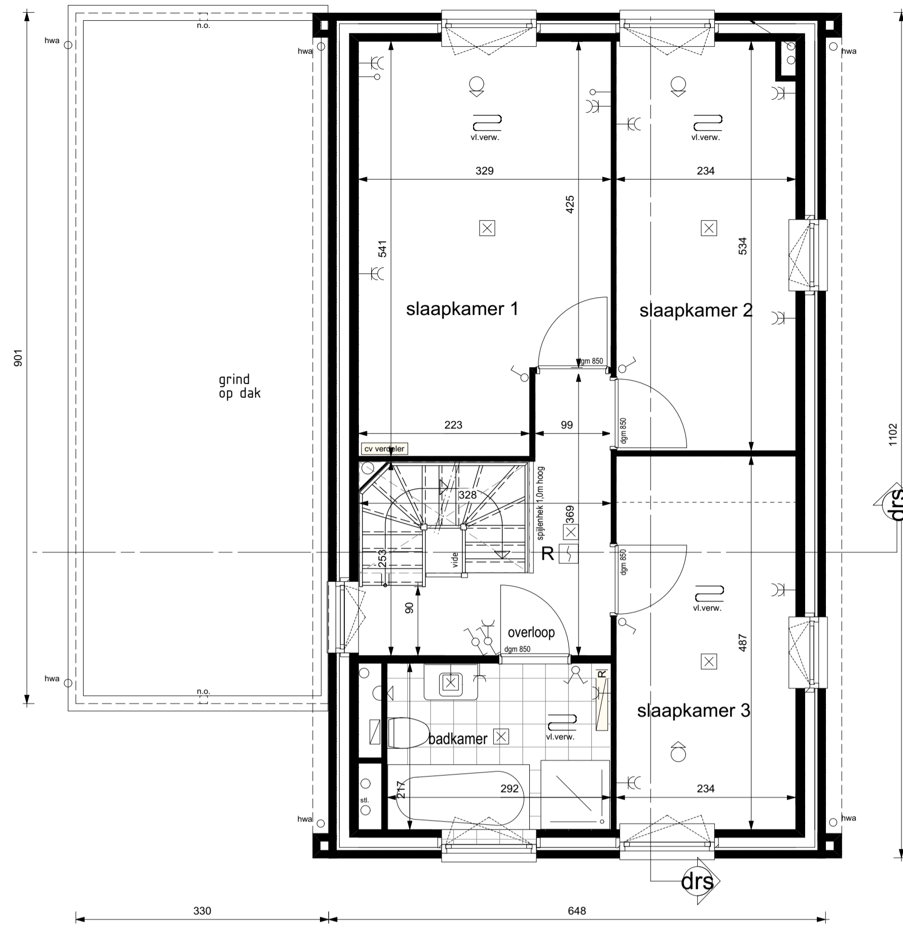
Verdieping
