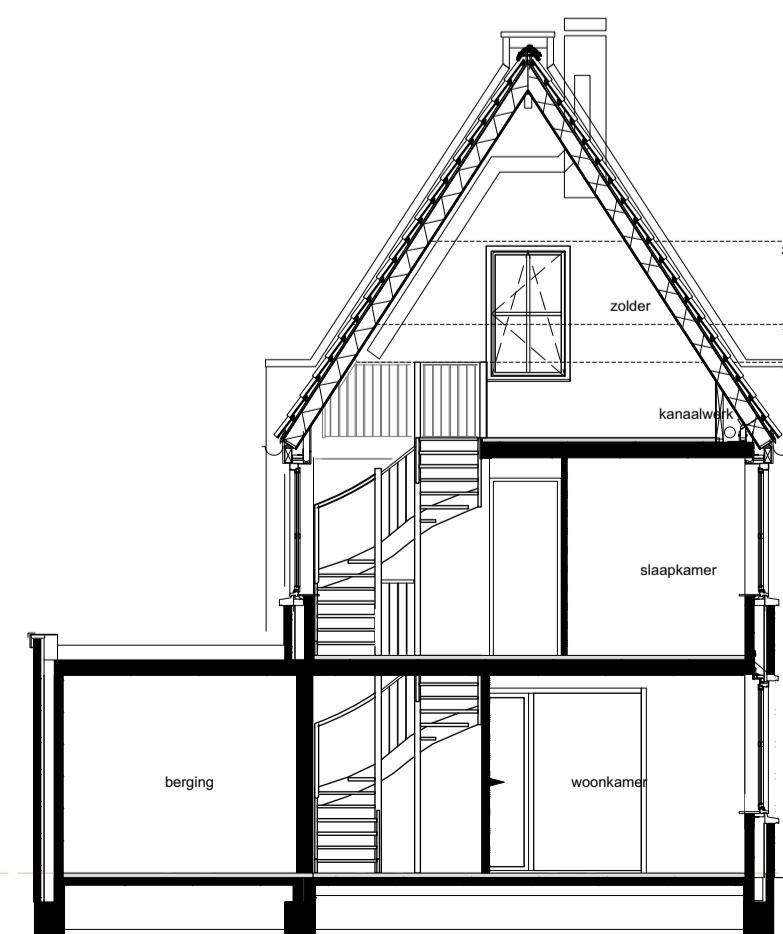
Doorsnede
