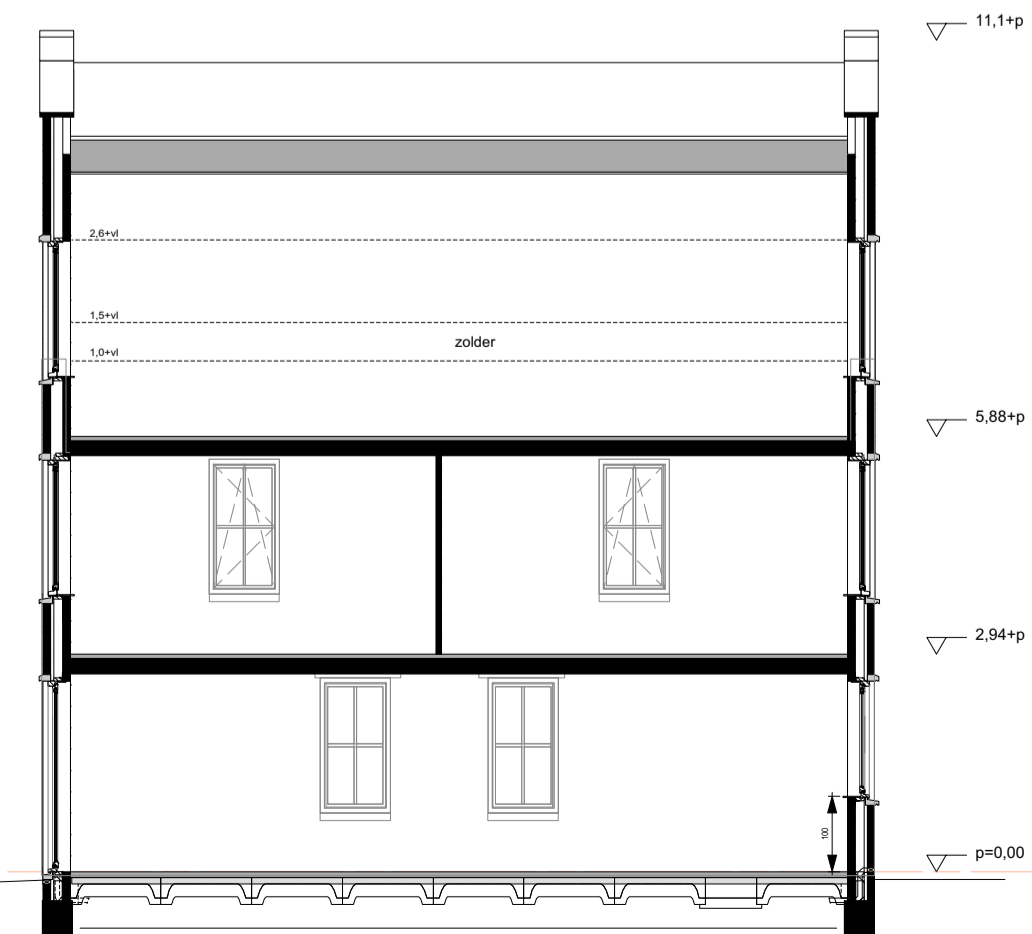
Doorsnede
