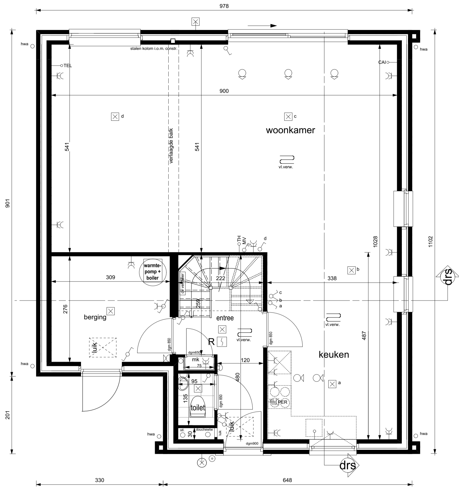
Begane Grond
