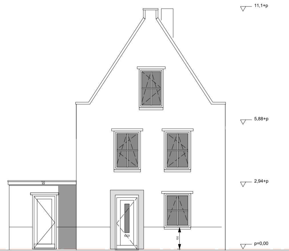
Voorgevel
