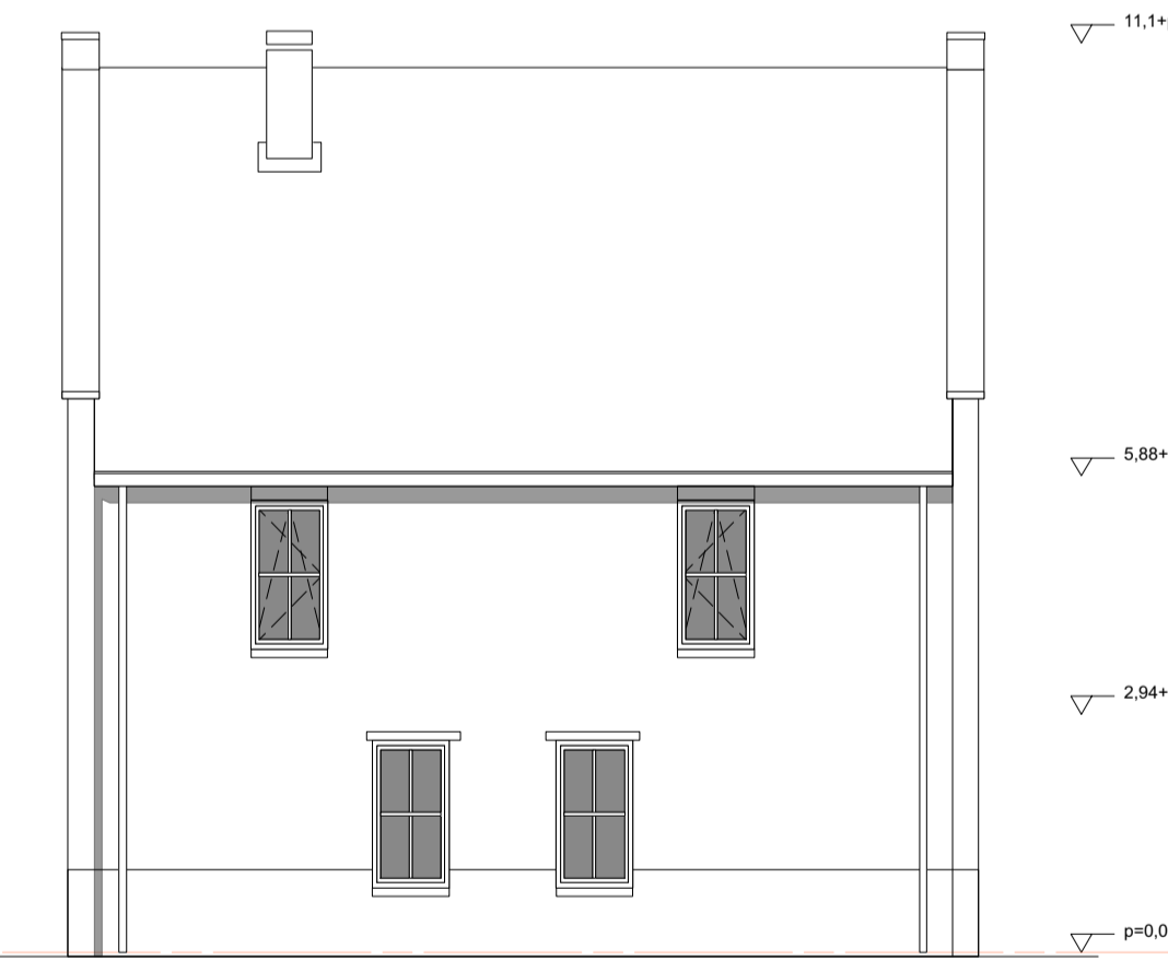
Zijgevel rechts
