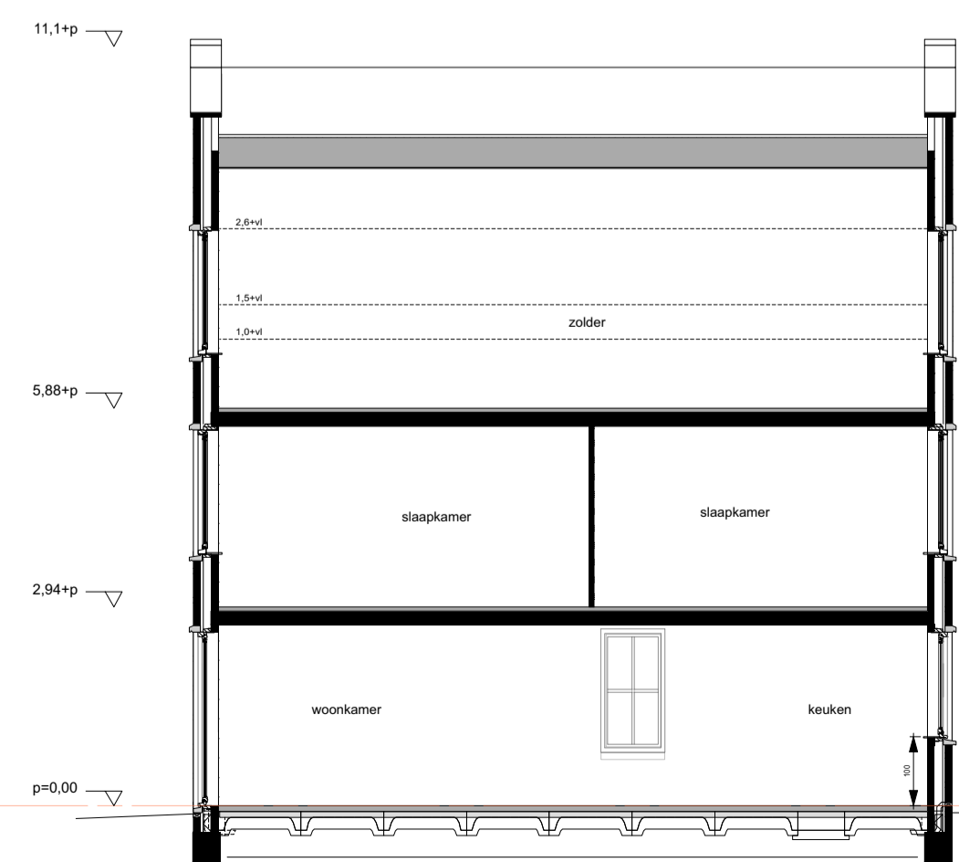
Doorsnede
