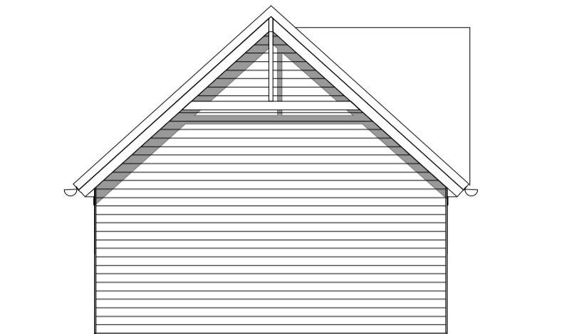
Zijgevel garage
