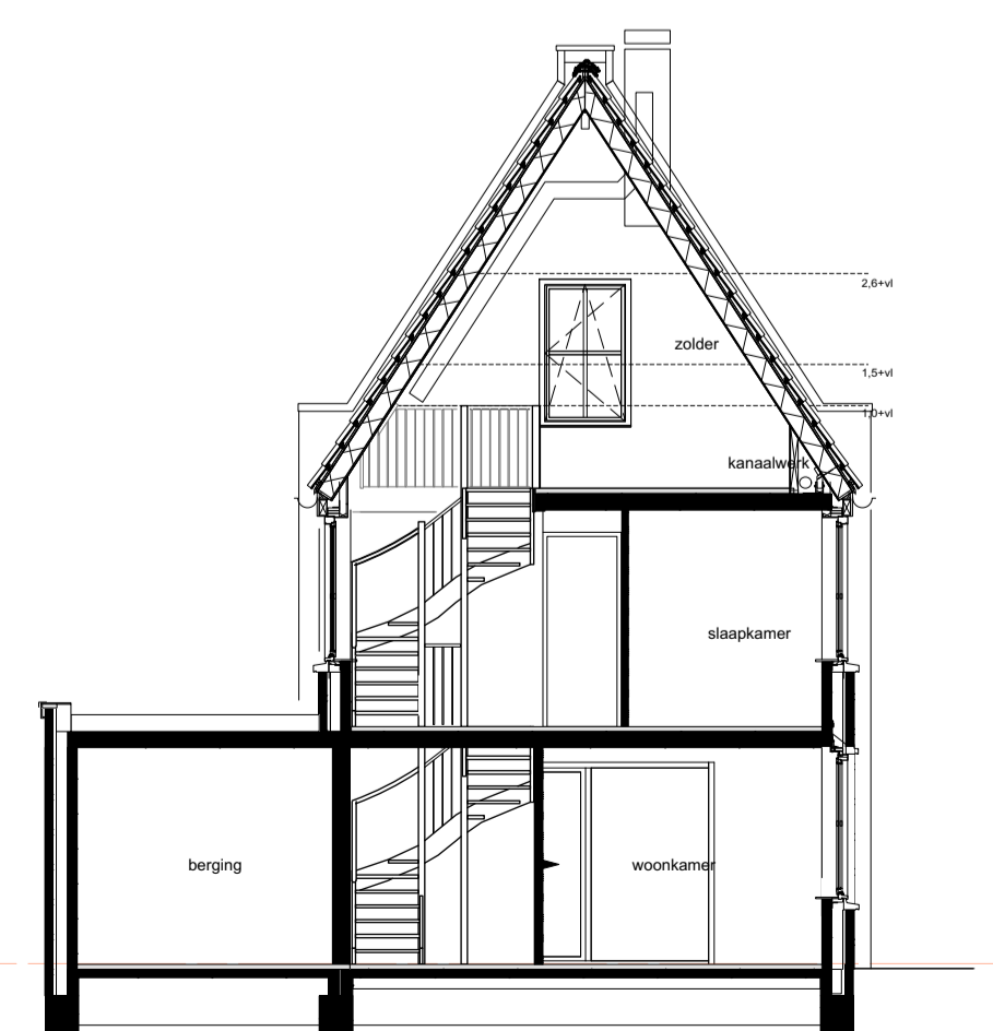
Doorsnede
