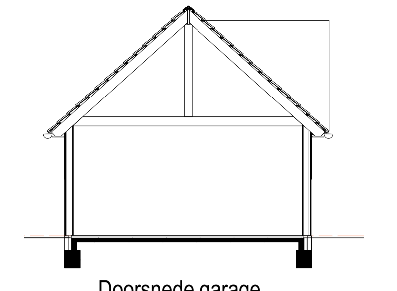
Doorsnede garage
